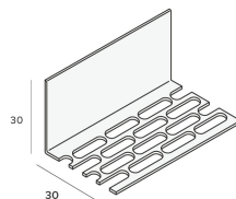
Geventileerd hoekprofiel nr. 0132
