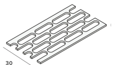
Geventileerd platprofiel nr. 1634
