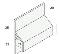
Trim/kraal aansluitprofiel nr. 2810
