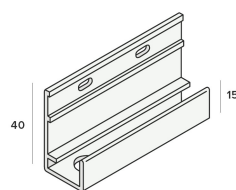
Omrandingsprofiel nr. 2809
