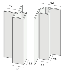
Uitwendig hoekprofiel nr. 2828
