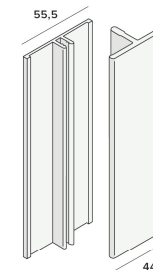
Basis verbindingsprofiel nr. 2805
