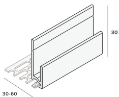
Inhaak startprofiel nr. 2808
