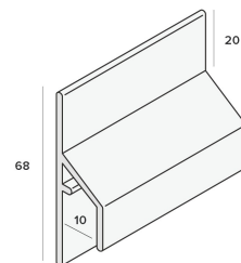
Trim/kraal aansluitprofiel nr. 2843
