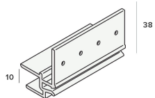
Montageprofielen 10 mm nr. 2867
