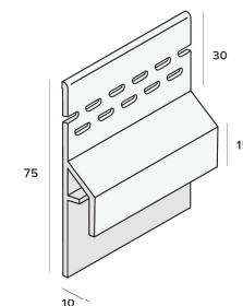
Trim ventilatie dakrand nr. 2833
