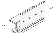
Montageprofielen 17 mm nr. 2877
